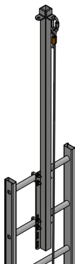
Extensión recta a fijaren los peldaños, altura 1500
