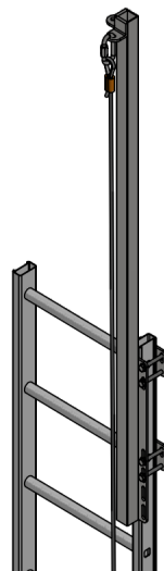
Extensión recta a fijar en el montante lateral, altura 1500
