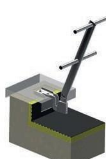
Fissaggio sotto scossalina (velletta isolata) montante inclinato
