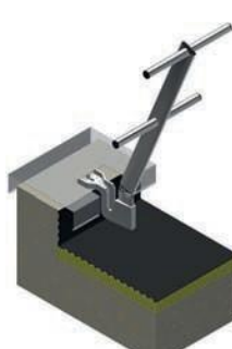
Fissaggio sotto scossalina standard montante inclinato
